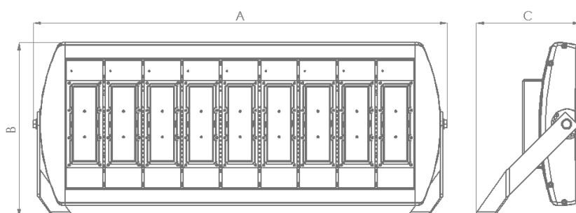
LENTE 30 x 30°
